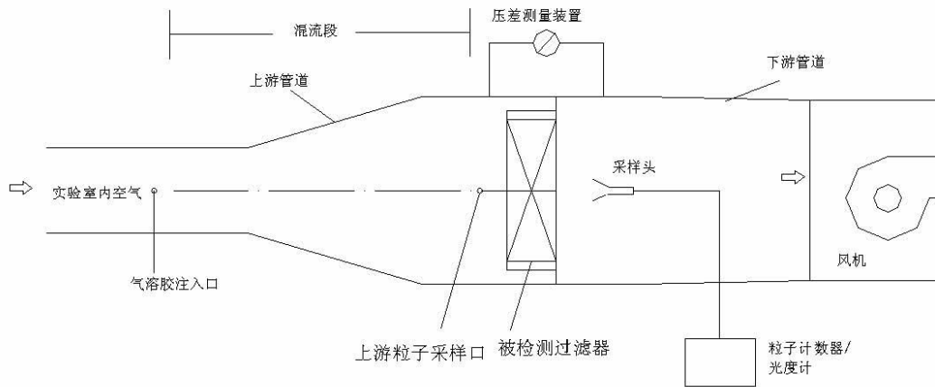
图1 扫描检漏法检测示意图
